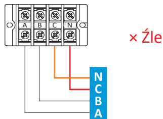
LISTWA ZACISKOWA
