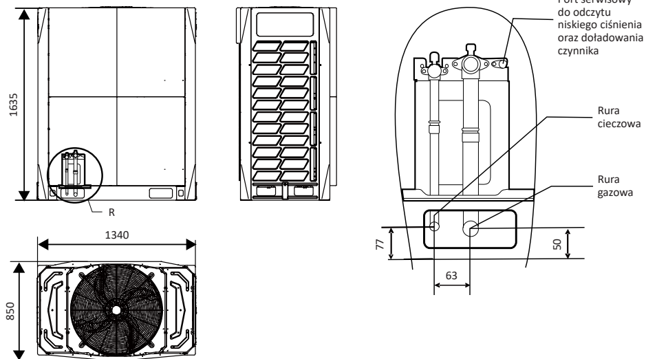
Średnice rur przyłączeniowych dla agregatu [mm]
