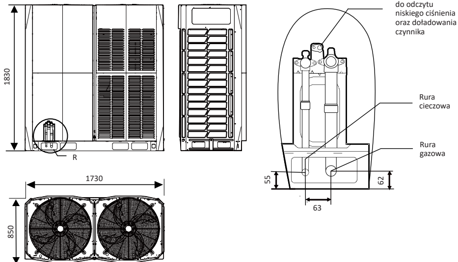
Średnice rur przyłączeniowych dla agregatów [mm]
