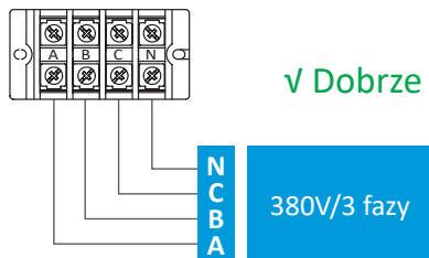
LISTWA ZACISKOWA
